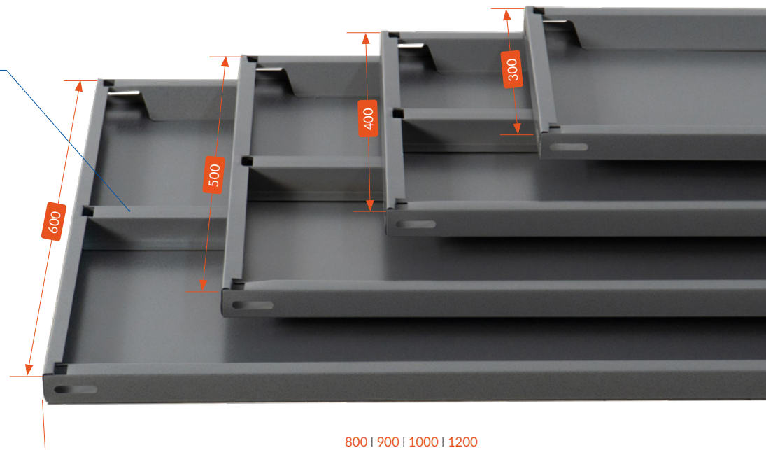
Renforts longitudinaux
